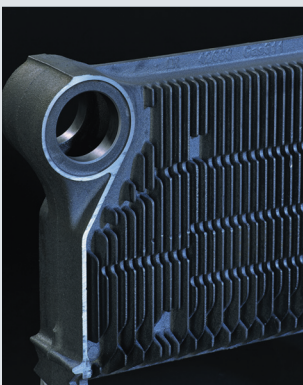
Теплообменные поверхности из эвтектического серого чугуна
